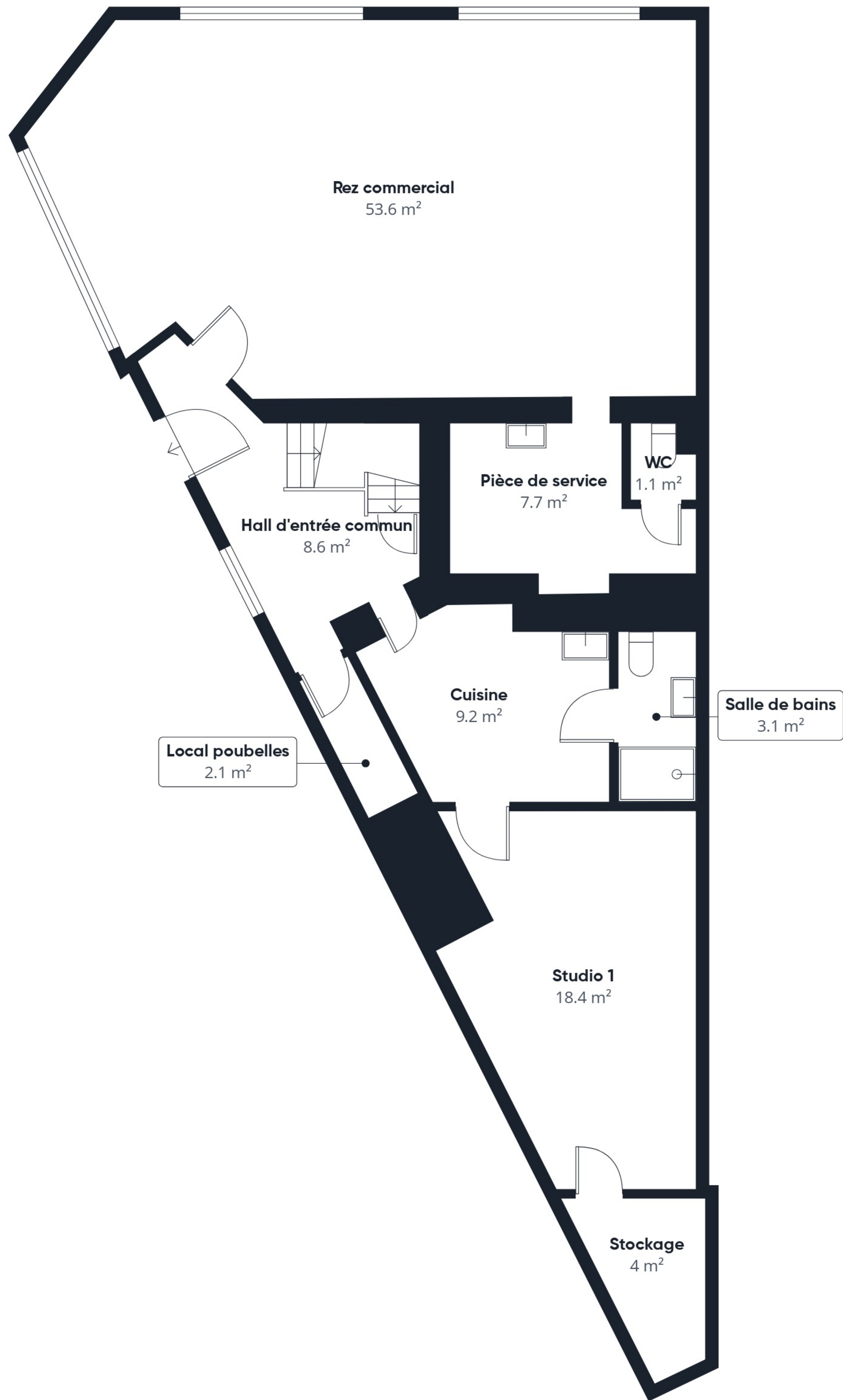
Niveau 0
